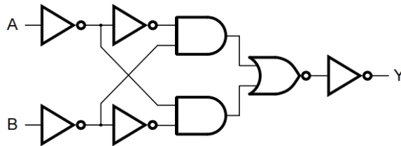
图 3 逻辑框图
